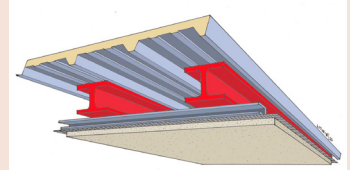
TOITURE ISOLÉE
