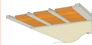
PLANCHER HOURDIS BRIQUE POUTRELLE BÉTON
